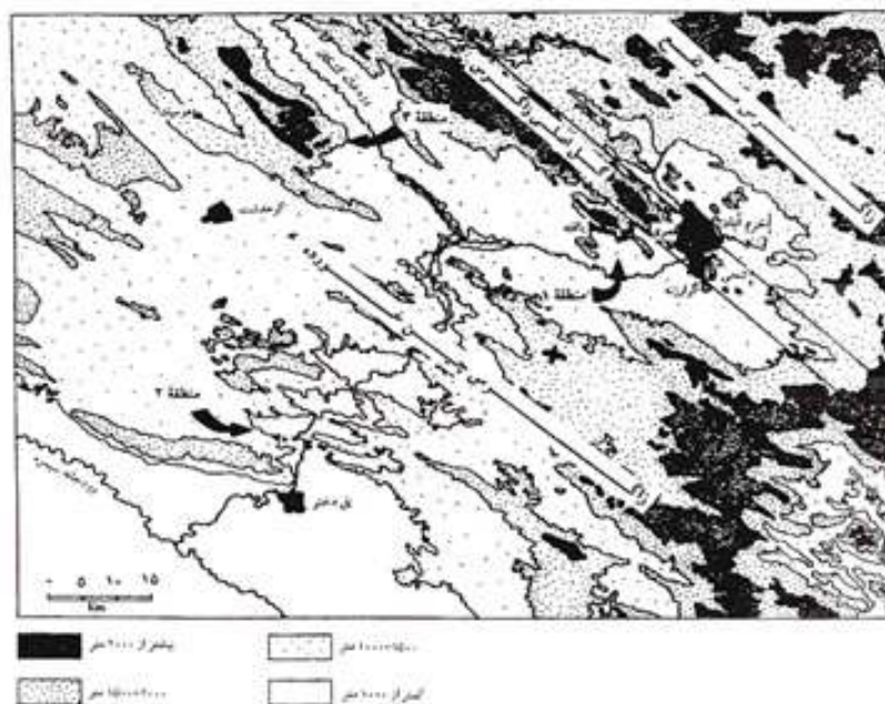
نقشه ۱- نقشه مناطق زمین‌شناسی، ناهمواری‌ها و پراکندگی محوطه‌های پارینه‌سنگی در استان لرستان (دایره‌های توپر: محوطه‌های نویافته؛ دایره‌های توخالی: محوطه‌های کاوش‌شده)
